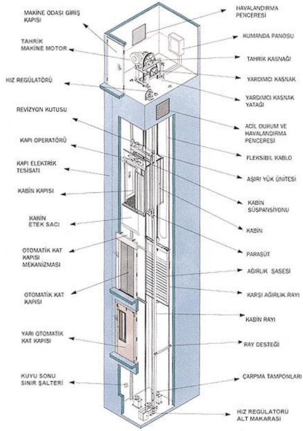
ASANSÖR GENEL MONTAJ RESMİ - ŞEKİL 2.1.1
